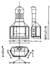
DK-3-AS HÁRSZÉKES TŰZTÉR KÉRDŐJELES VÁLTOZATOKAL KÉRDŐJELES VÁLTOZATOKAL
