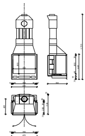
DK-3-AS HÁRSZÉKES TŰZTÉR KÉRDŐJELES VÁLTOZATOKAL KÉRDŐJELES VÁLTOZATOKAL
