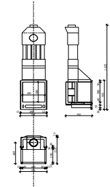
DK-1-ES HÁRSZÁRÚ TÍPUSÚ TÚZTÉR SPEJLI DALSÓ NYITÁSI ÁLLÁSŰZEL SPEJLI DALSÓ NYITÁSI ÁLLÁSŰZEL
